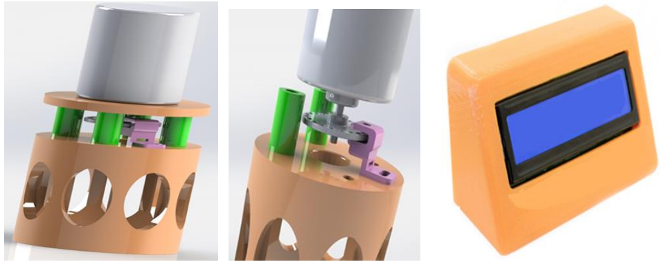
Макет ротационного датчика вязкости
