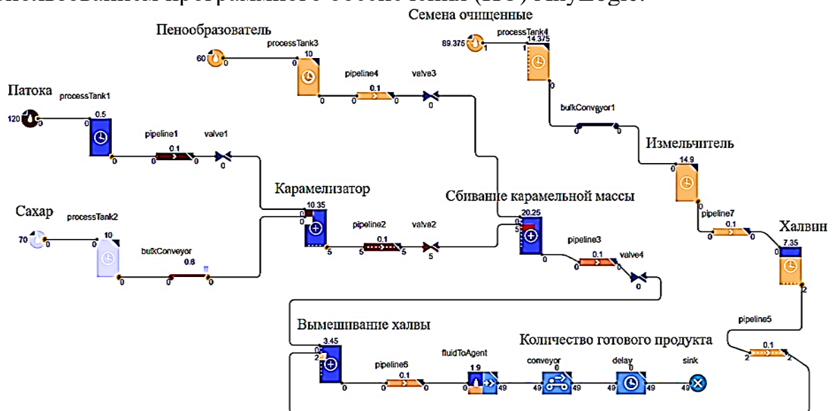
Рисунок 4.1. Имитационная модель процесса производства халвы
