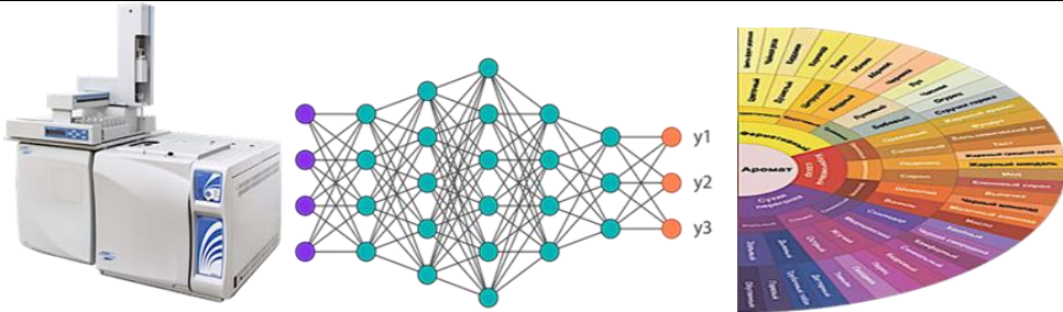
Схема автоматического контроля запаха КП с использованием НСТ
