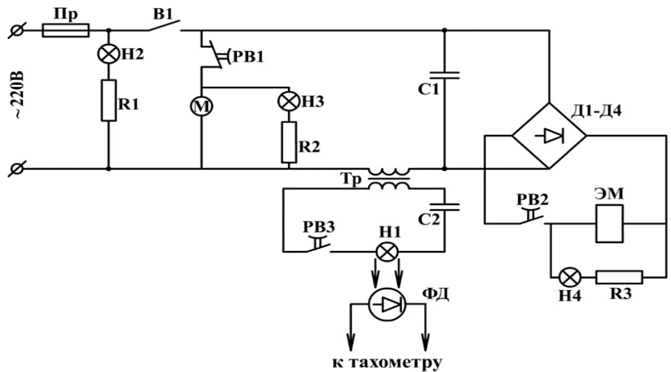
ПЭС датчика вязкости ротационного цифрового вискозиметра
