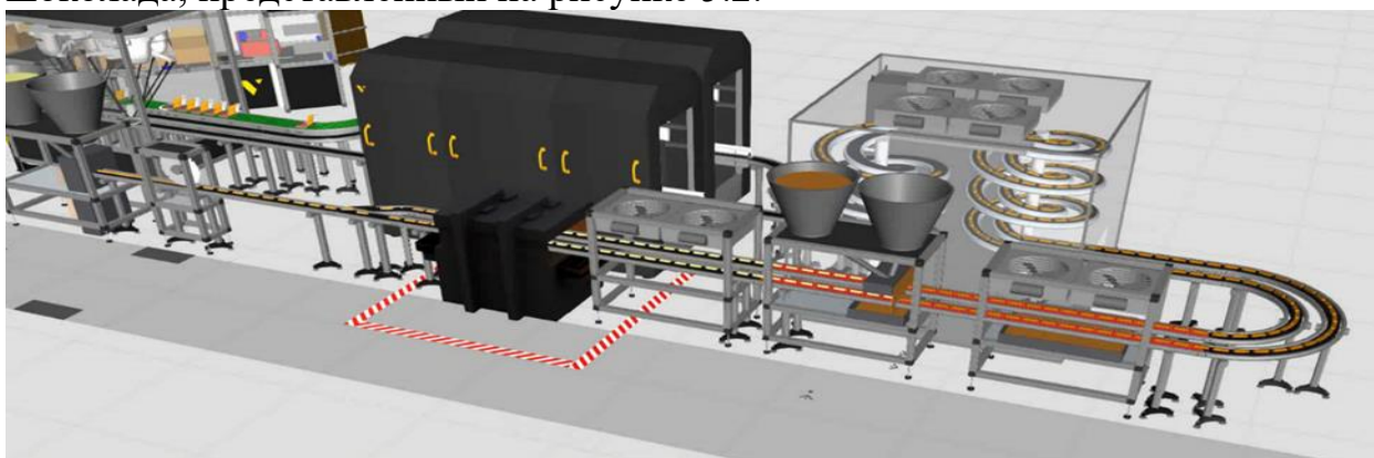
Рисунок 5.2 - Цифровой двойник ТП производства шоколада
