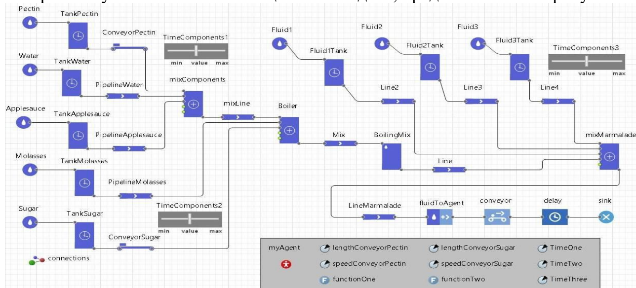
Рисунок 4.2 - Мультиагентная имитационная модель процесса производства мармеладных конфет
