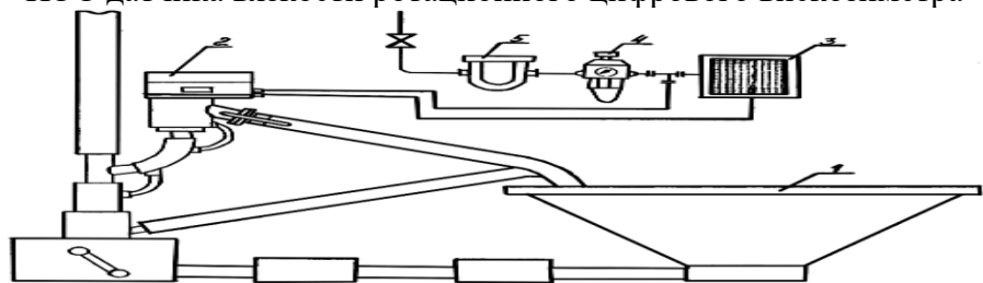
Схема установки автоматического вискозиметра
