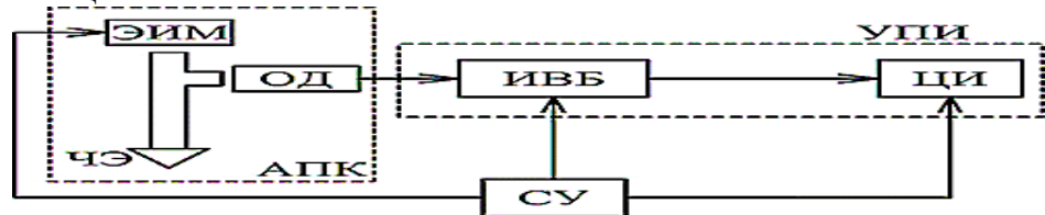
Структурная схема цифрового консистометра
